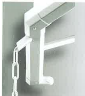
Entwässerung Mit Speier und Kette
